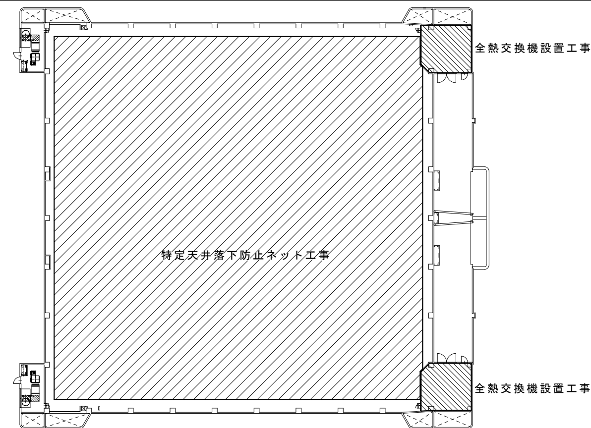
小屋裏兼天井伏図 S:1/500
