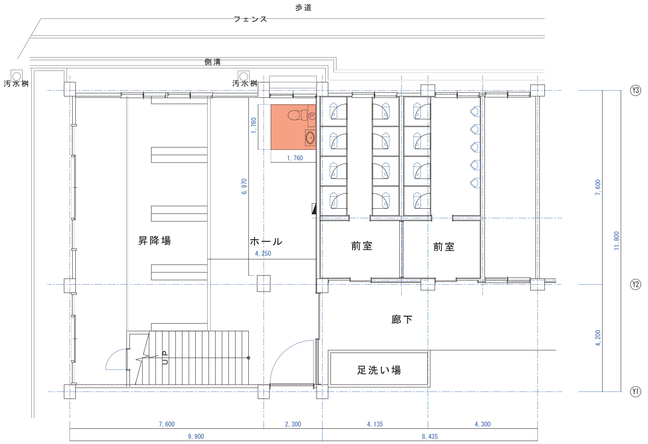
1 階 平面図
