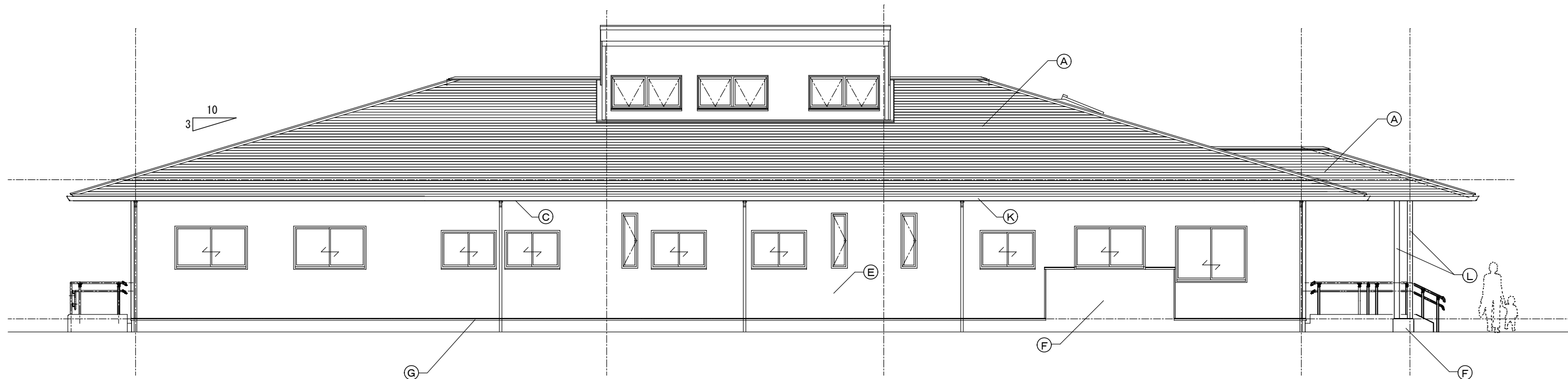
西側立面図 S=1:100
