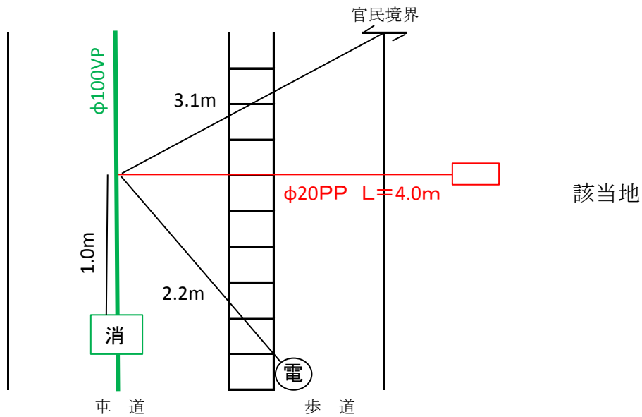
断面図 (縮尺/ )
