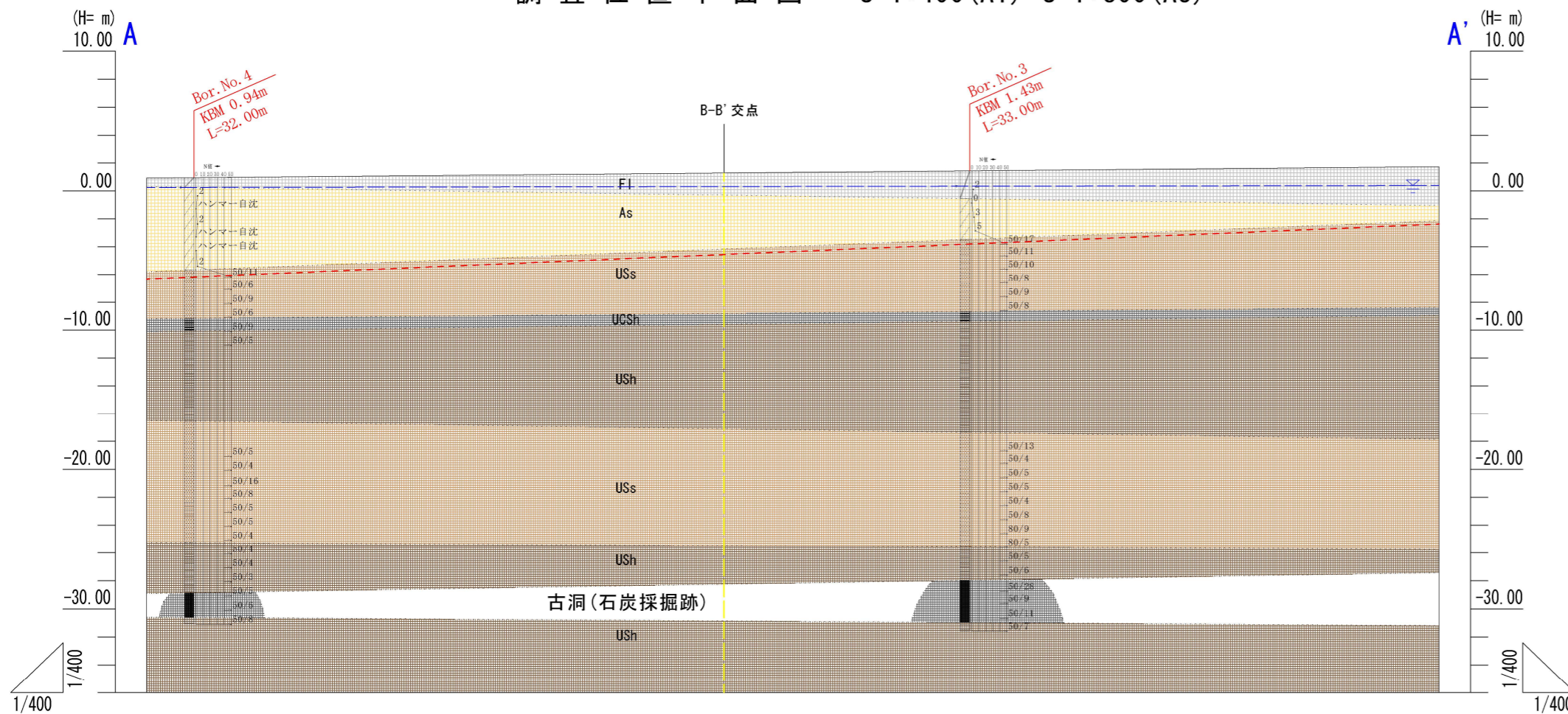
推定地質区分模式断面図 S=1:200(A1) S=1:400(A3)
