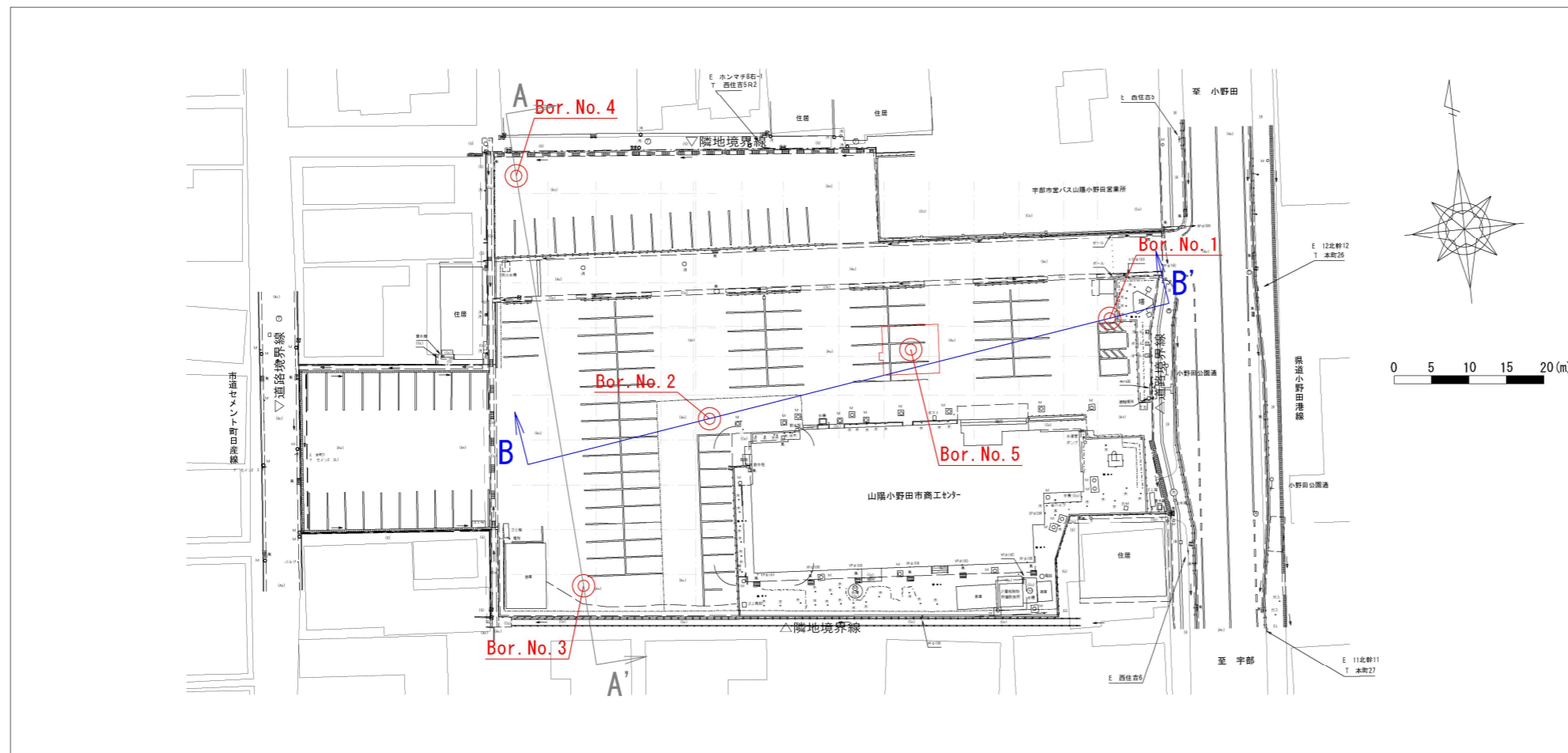
調査位置平面図 S=1:400(A1) S=1:800(A3)
