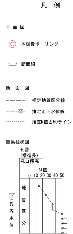
地質層序表
