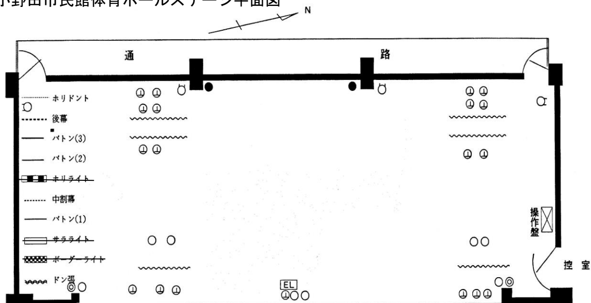
山陽小野田市民館体育ホールステージ平面図
