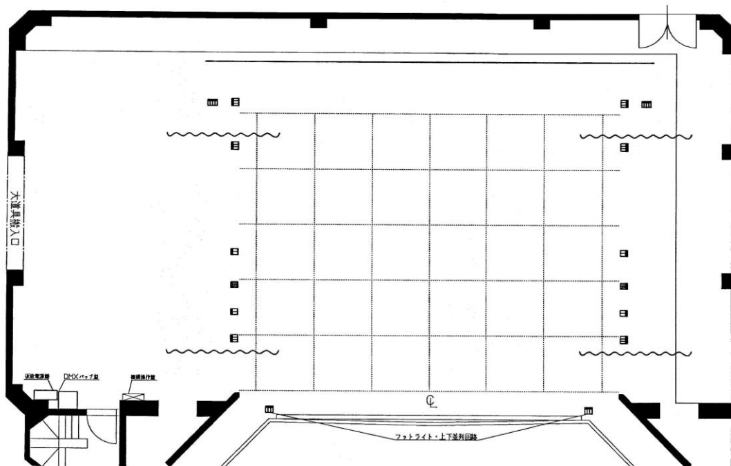
山陽小野田市民館文化ホールステージ平面図
