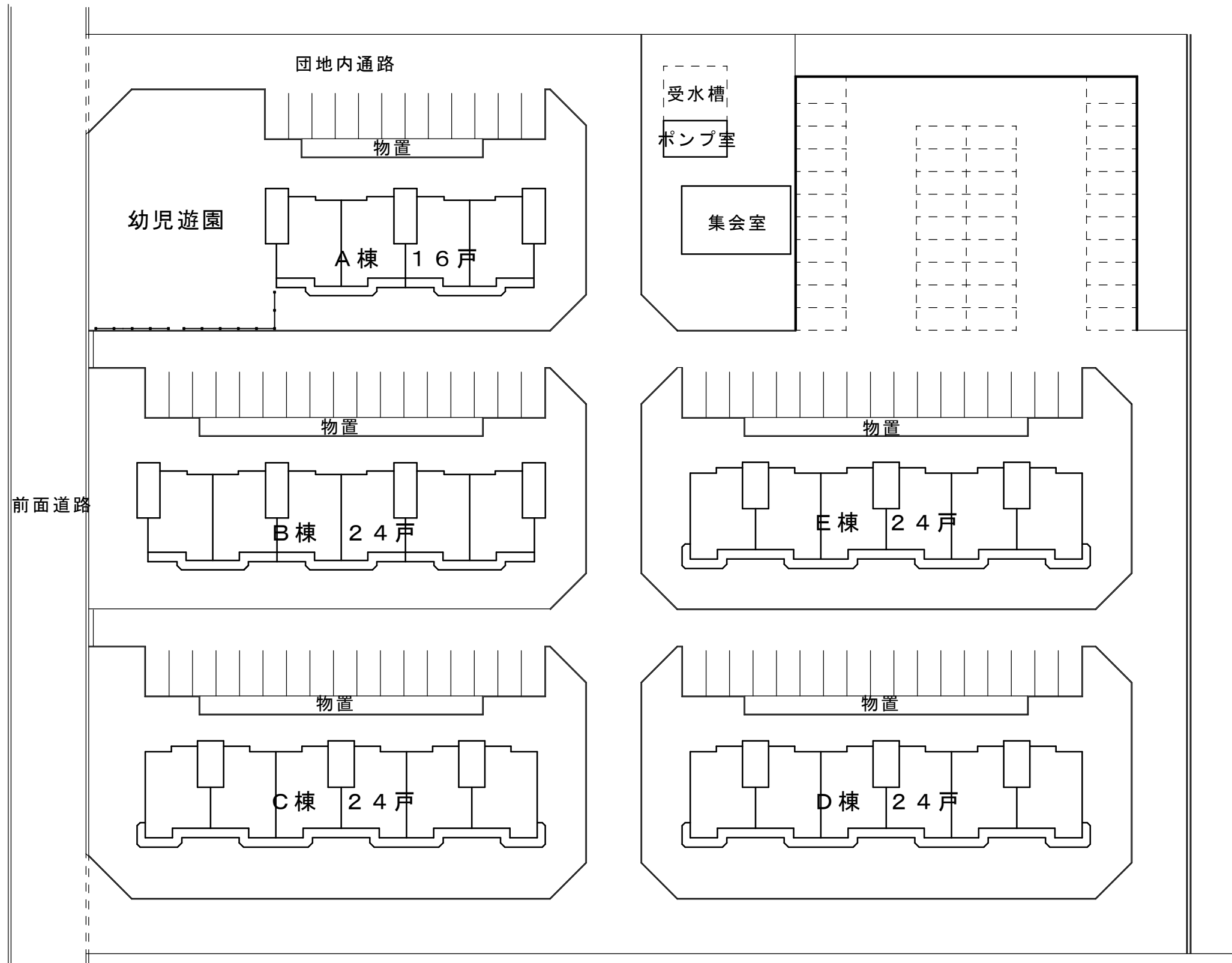
古開作団地 配置図 S=1/500
