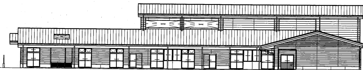
南側立面図
