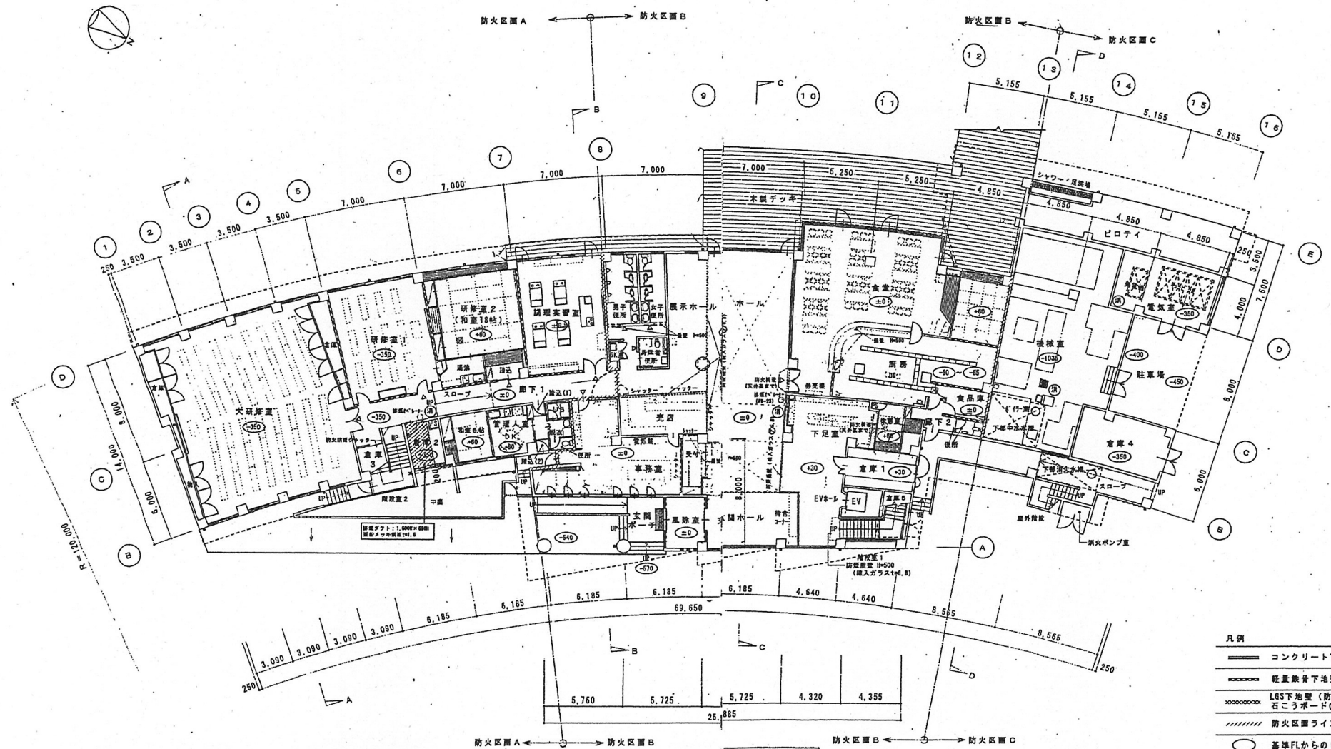
1階平面図
