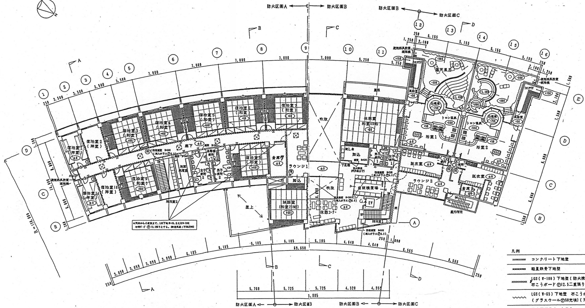
2階平面図
