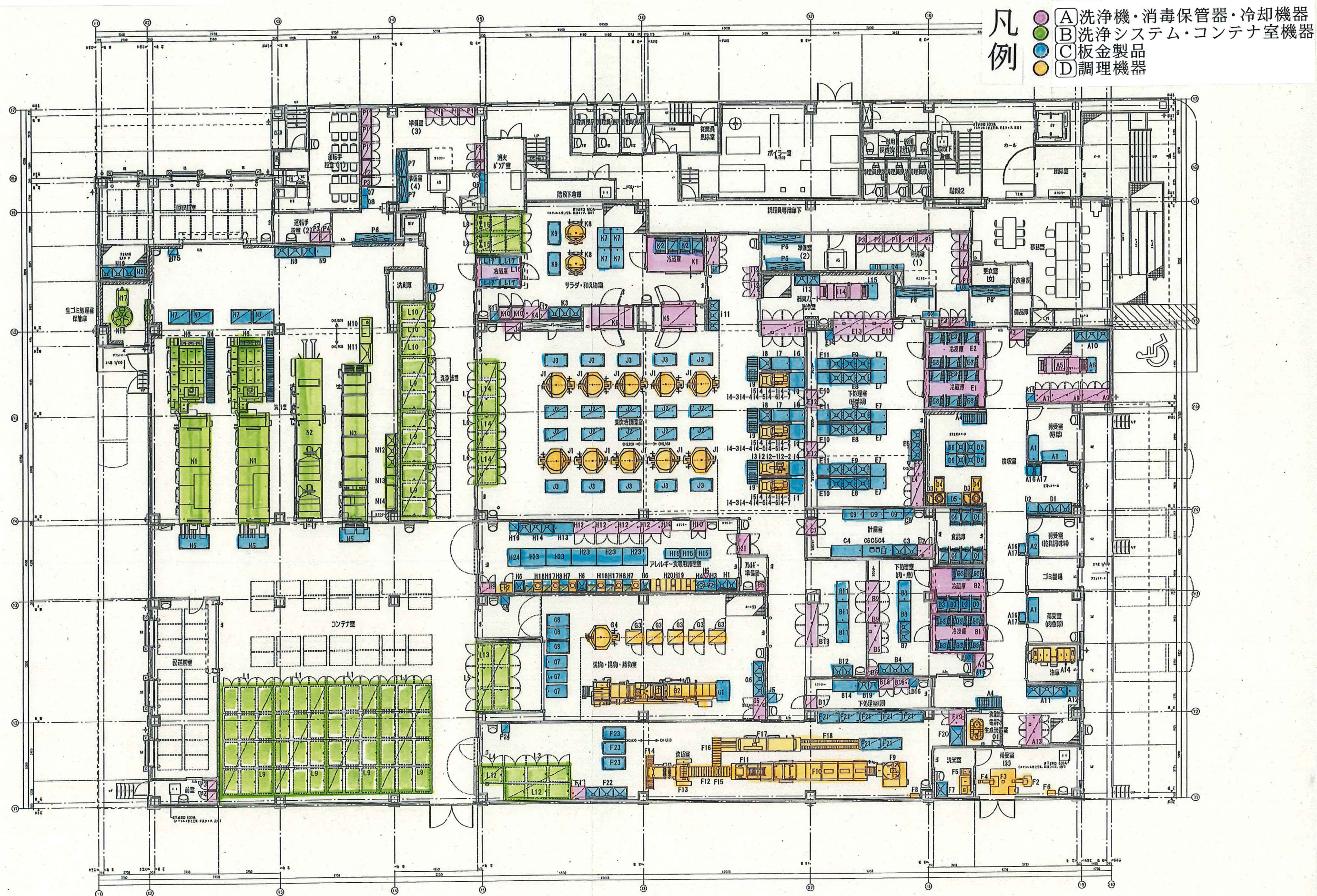
山陽小野田市学校給食センター厨房機器配置図
