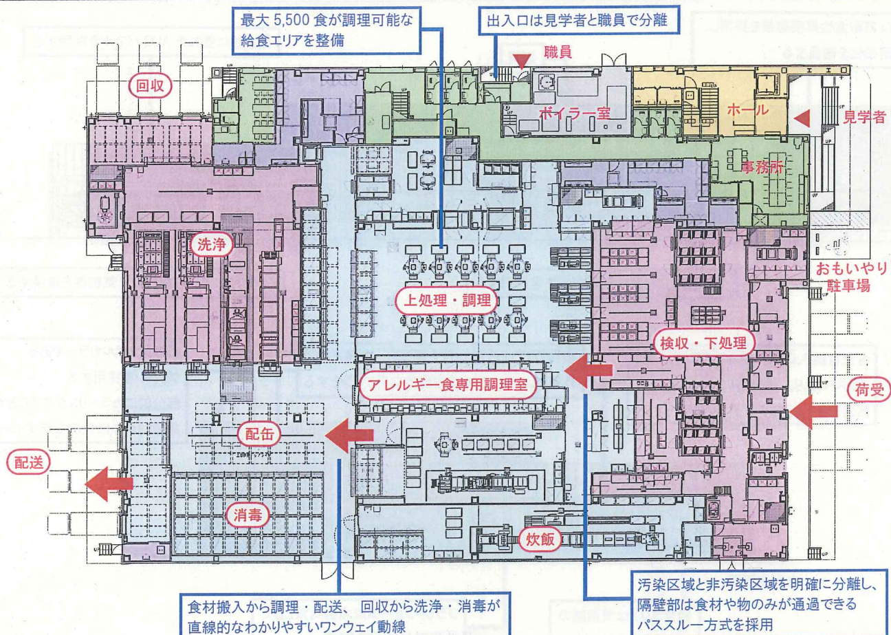
1階平面図
