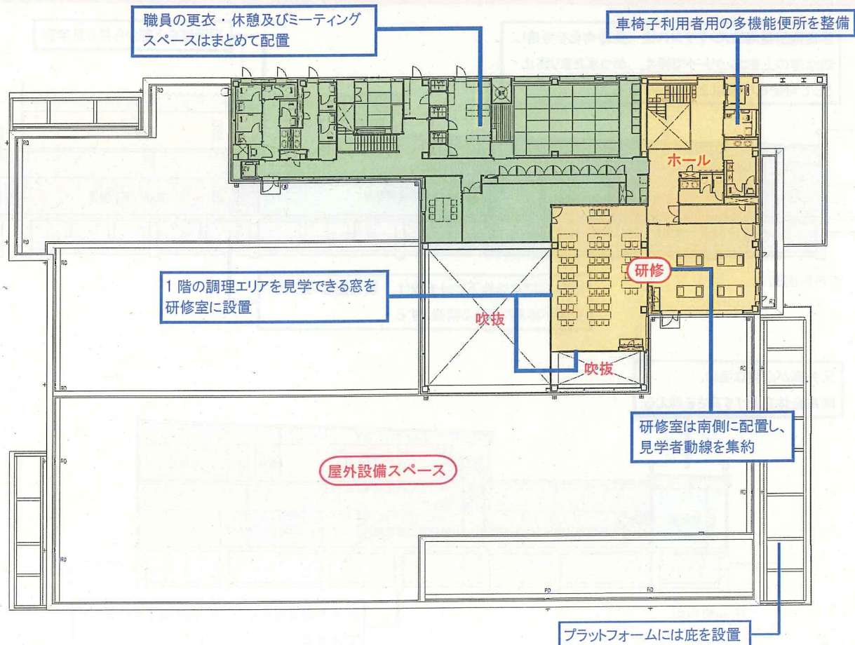
2階平面図
