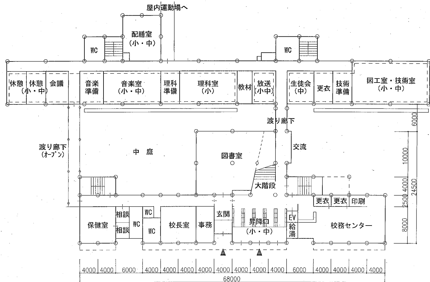
児童棟・生徒棟 1階平面図 1/500
