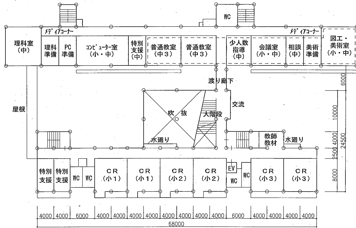
児童棟・生徒棟 2階平面図 1/500
