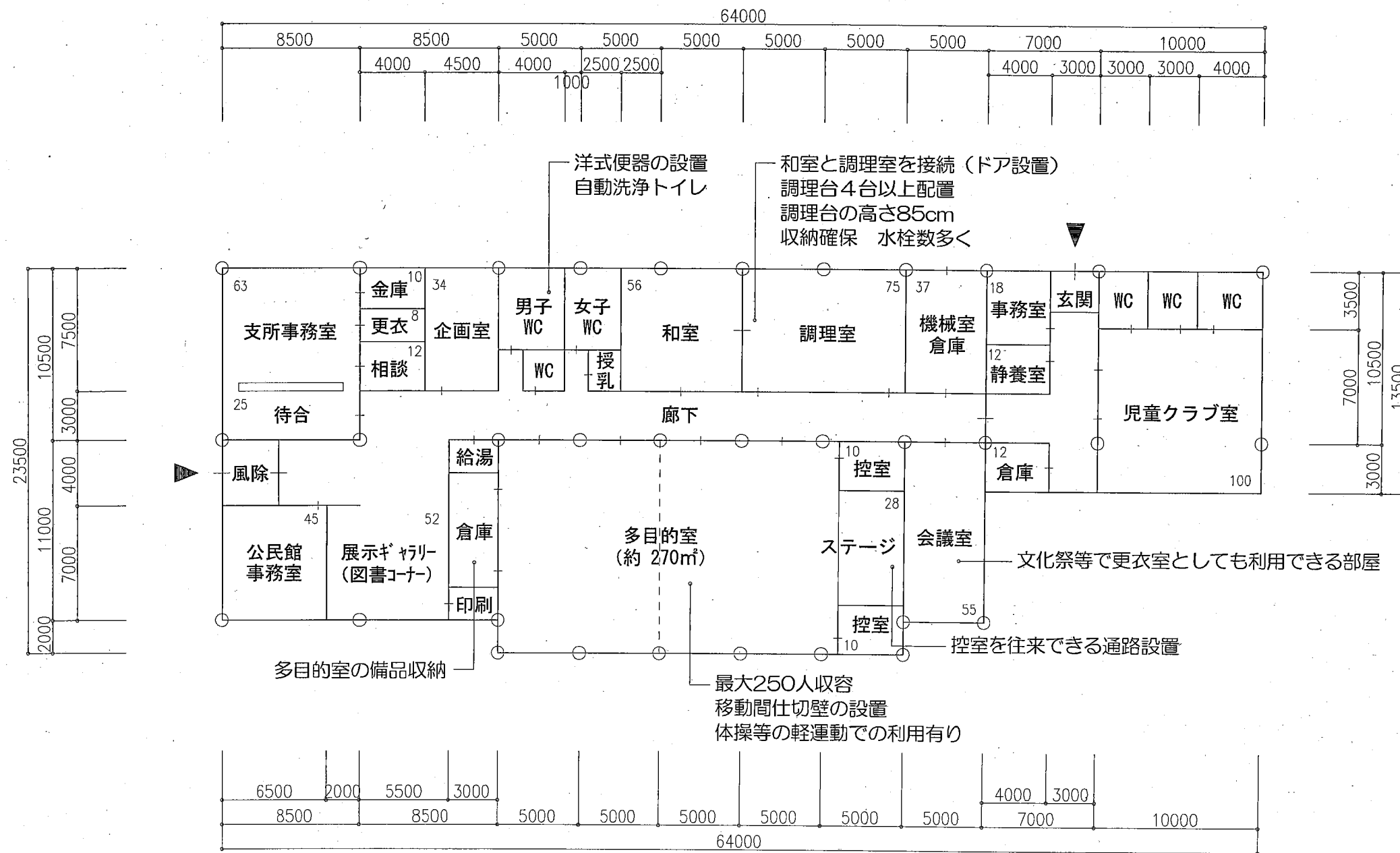
複合施設 1階平面図 1/300 計 1,290 m 2
