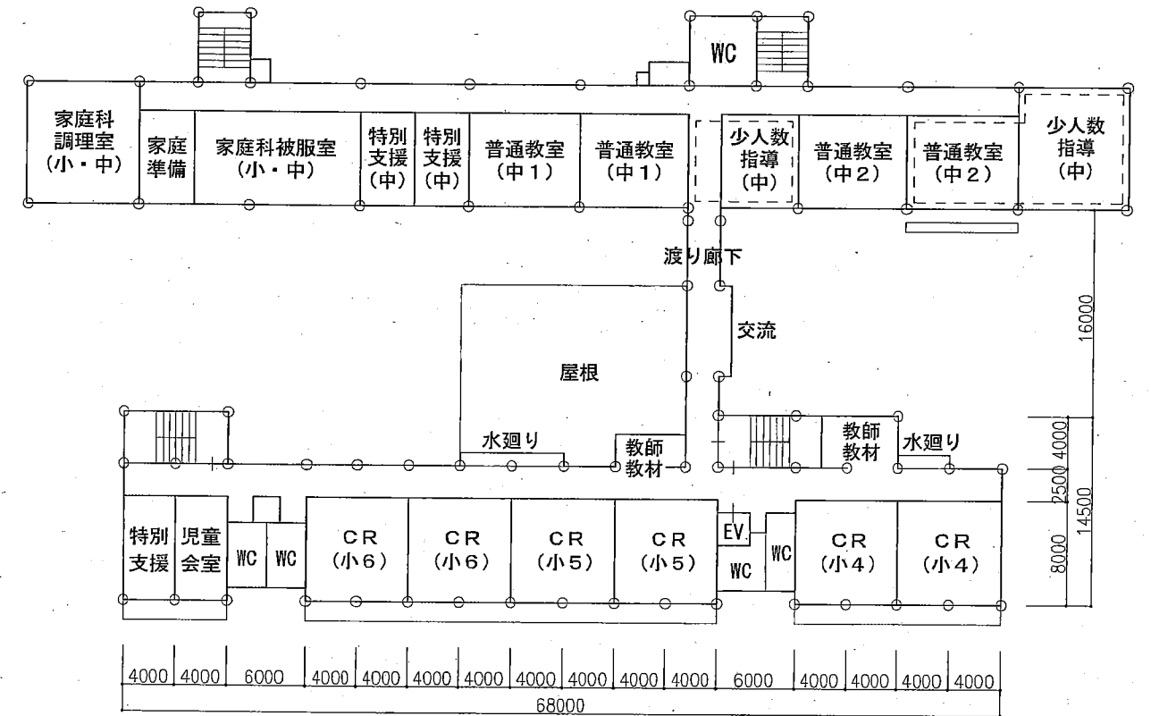
児童棟・生徒棟 3階平面図 1/500
