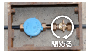
メーターボックス(左:メーター 右:止水栓)▲
