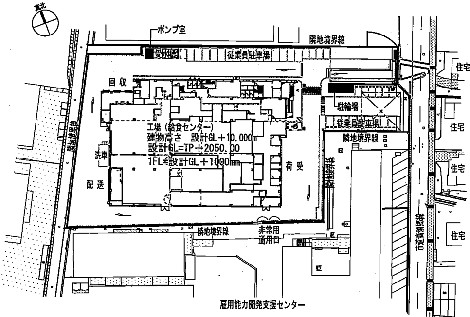
配置図
