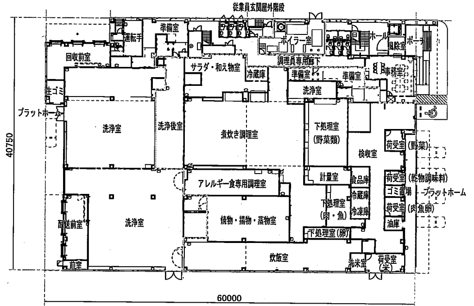
1階平面図
