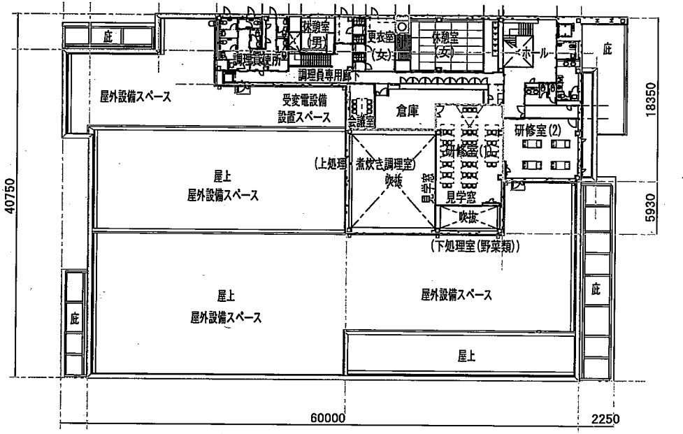
2階平面図
